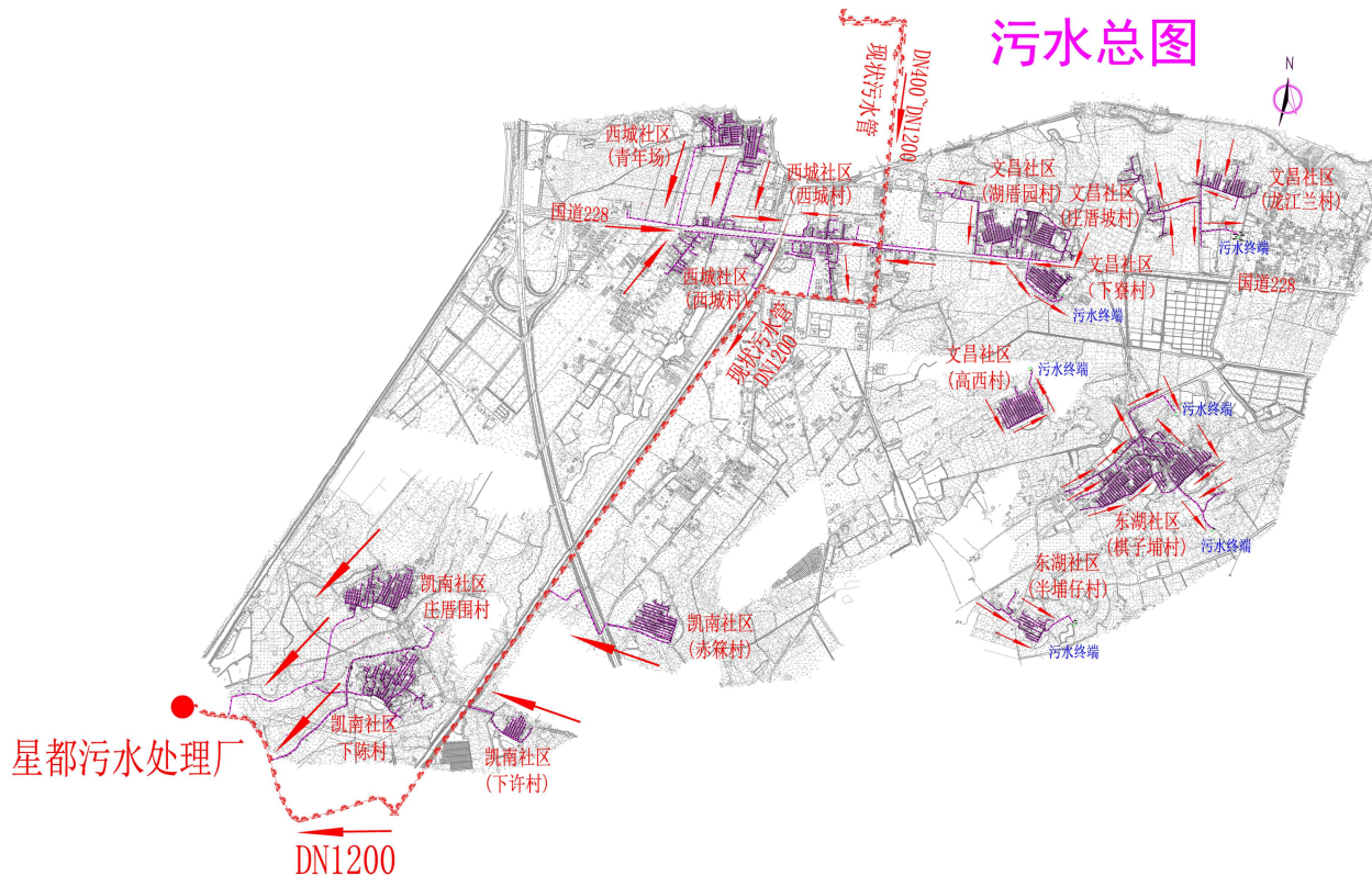
污水管网设计方案总体布置图
