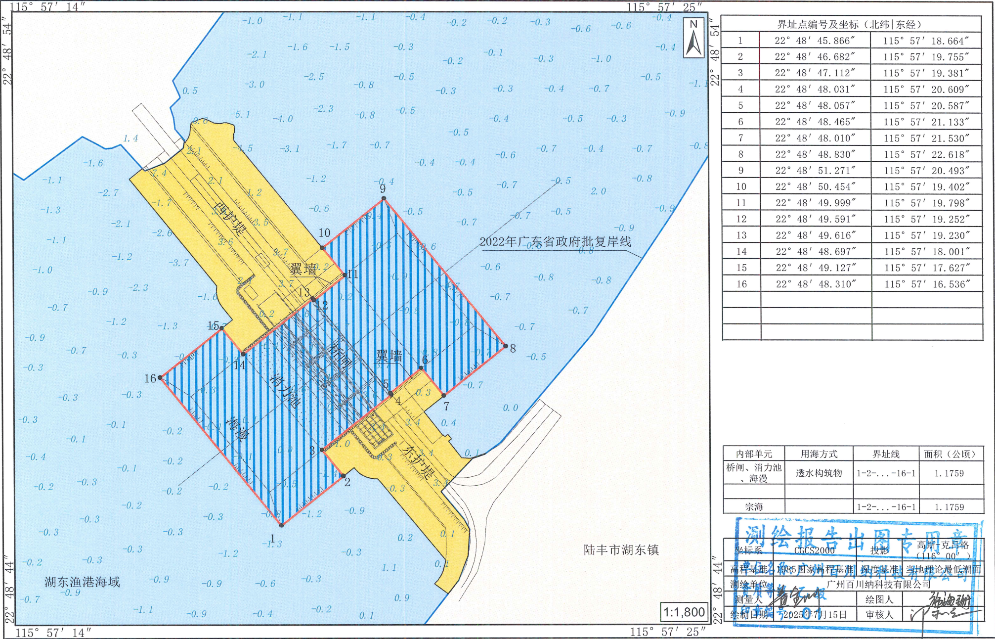
陆丰市湖东大桥桥闸重建工程（桥闸、消力池、海漫）宗海界址图
