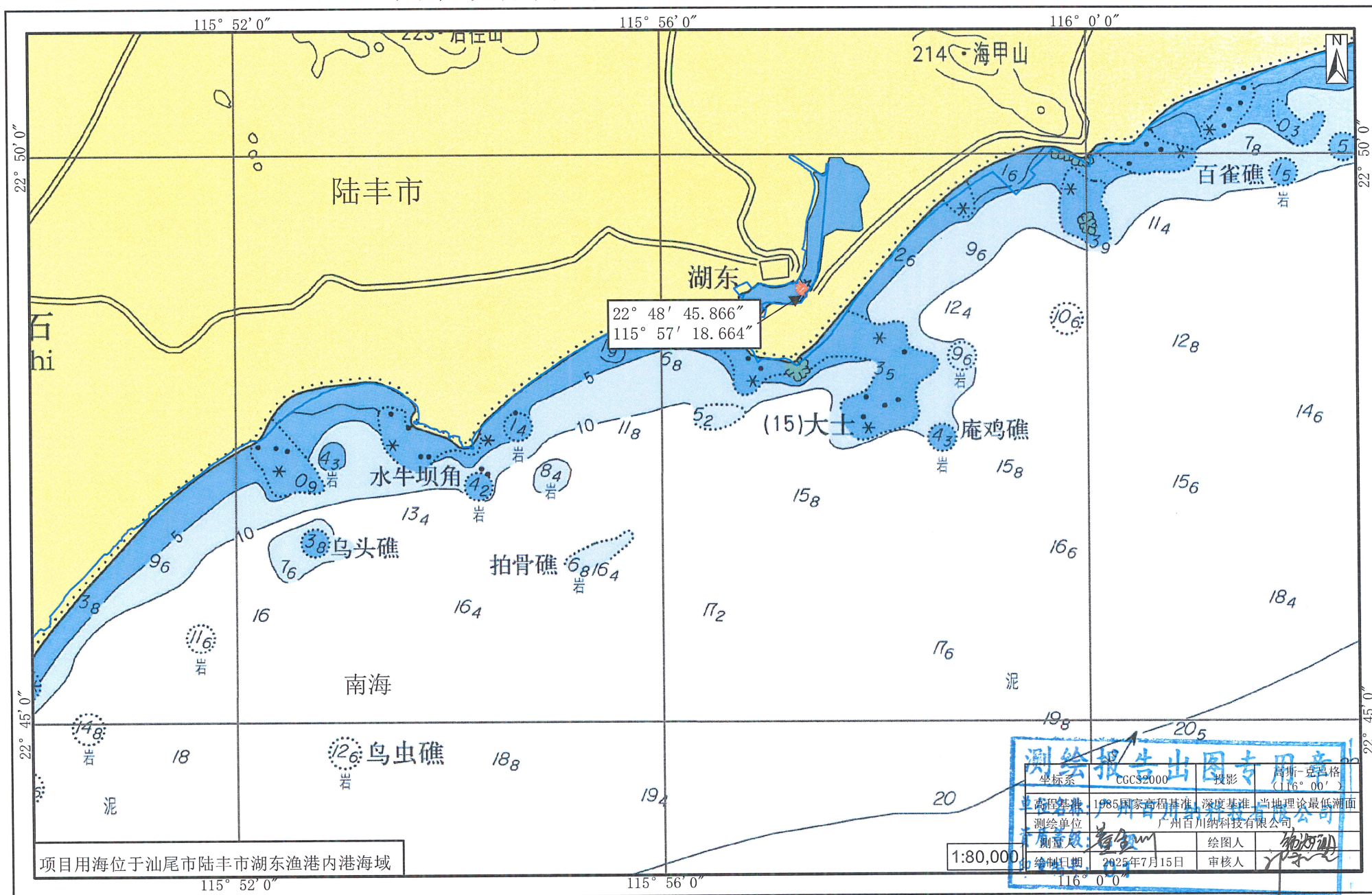
陆丰市湖东大桥桥闸重建工程宗海位置图
