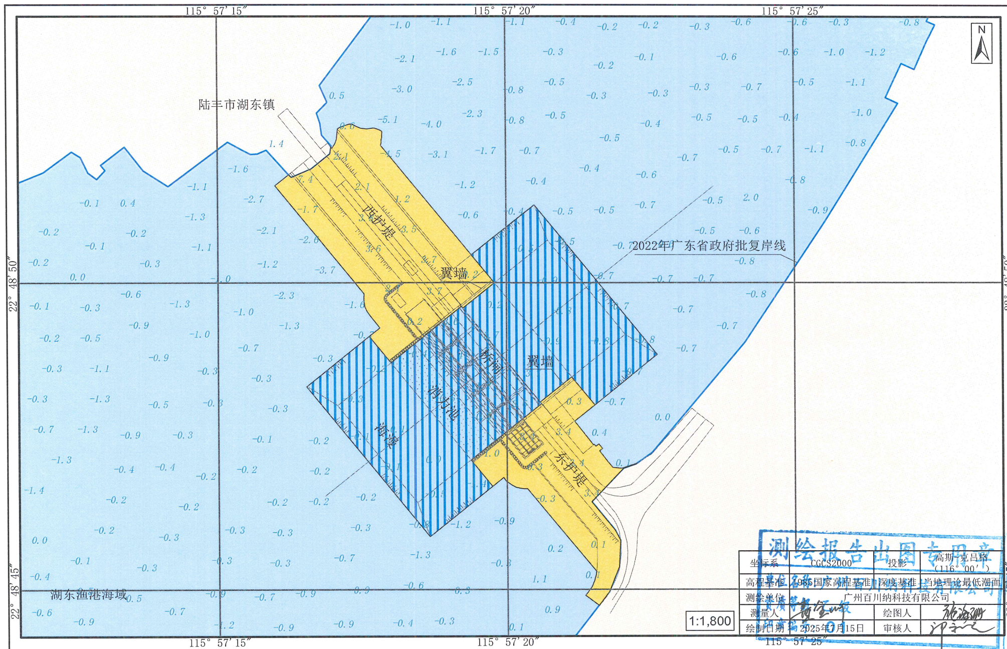
陆丰市湖东大桥桥闸重建工程宗海平面布置图
