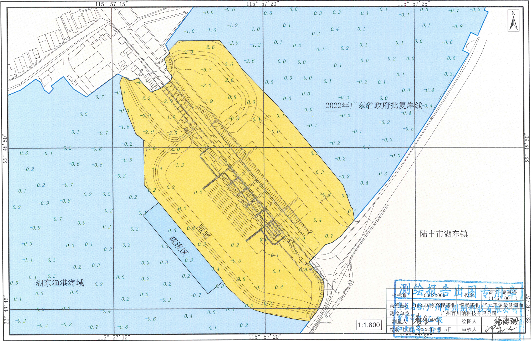
陆丰市湖东大桥桥闸重建工程（施工期）宗海平面布置图
