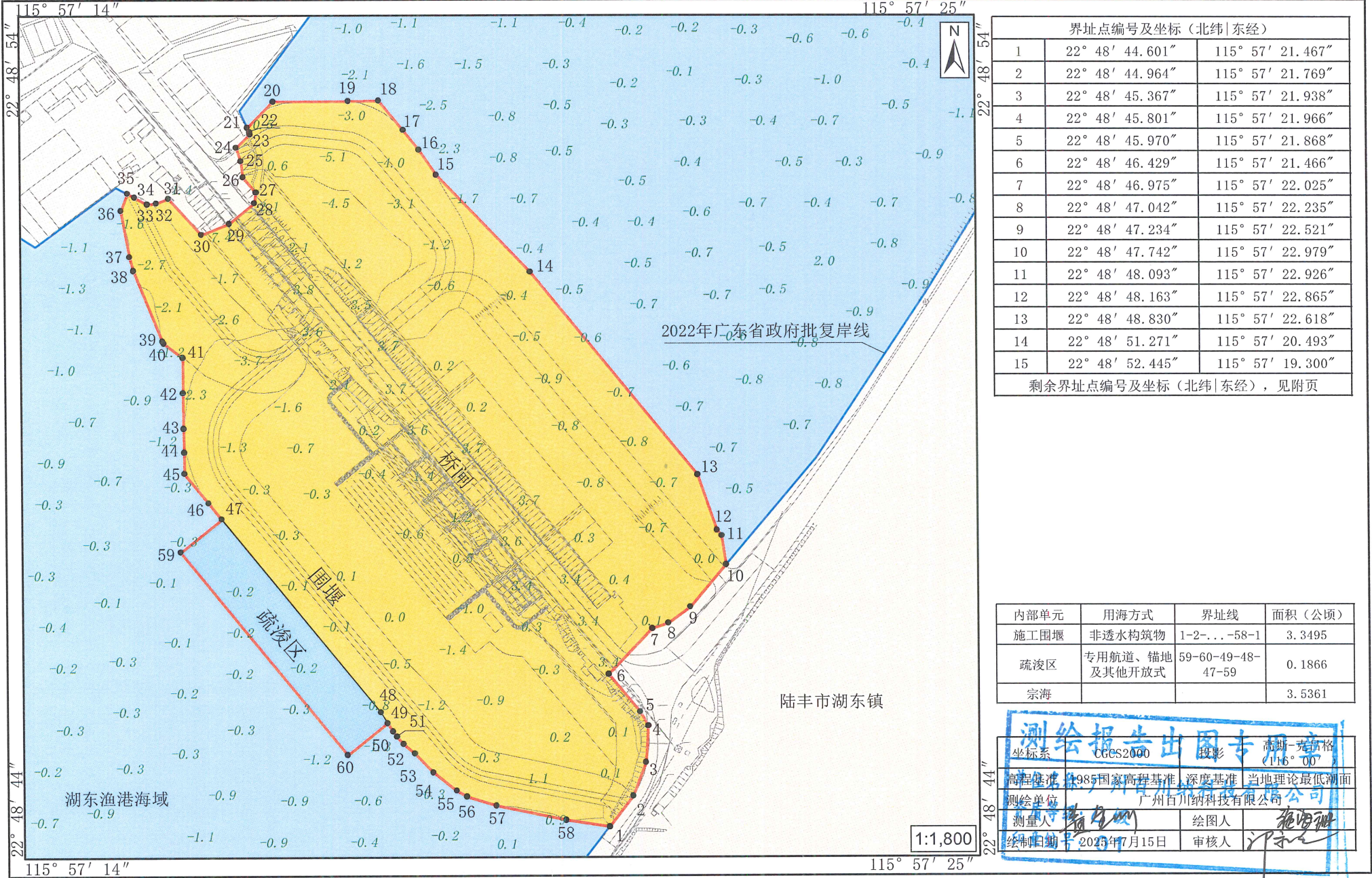
陆丰市湖东大桥桥闸重建工程（施工期）宗海界址图
