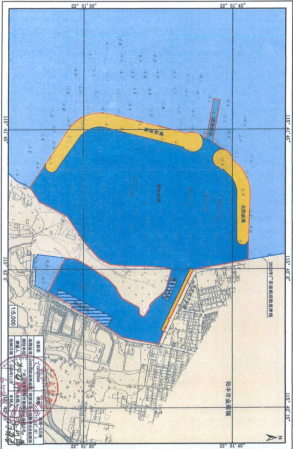
陆丰市金厢渔港建设项目宗海平面布置图
