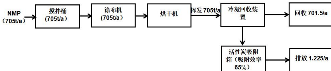
图 4-1 NMP 物料平衡图
