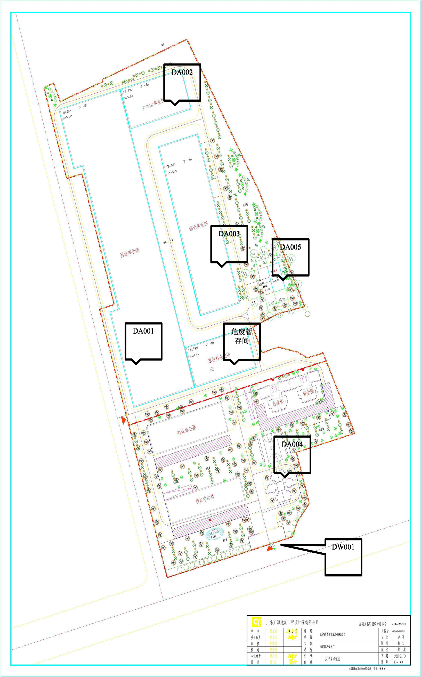
附图 4 项目总平面图
