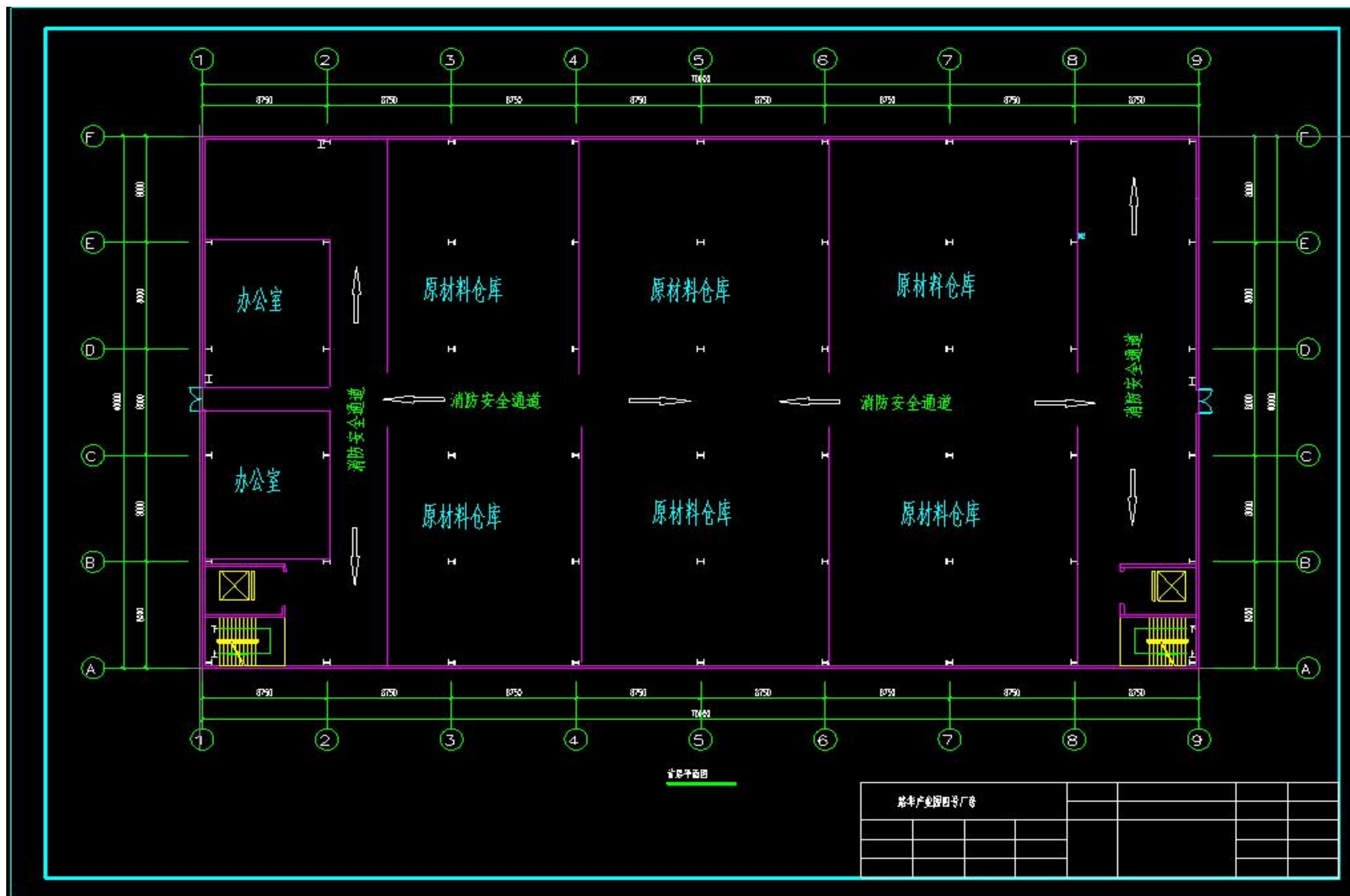
附图 20 车间四二层平面图
