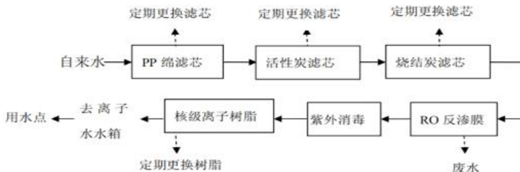
图 2-5 纯水制备生产工艺流程及污染物产生点位图
