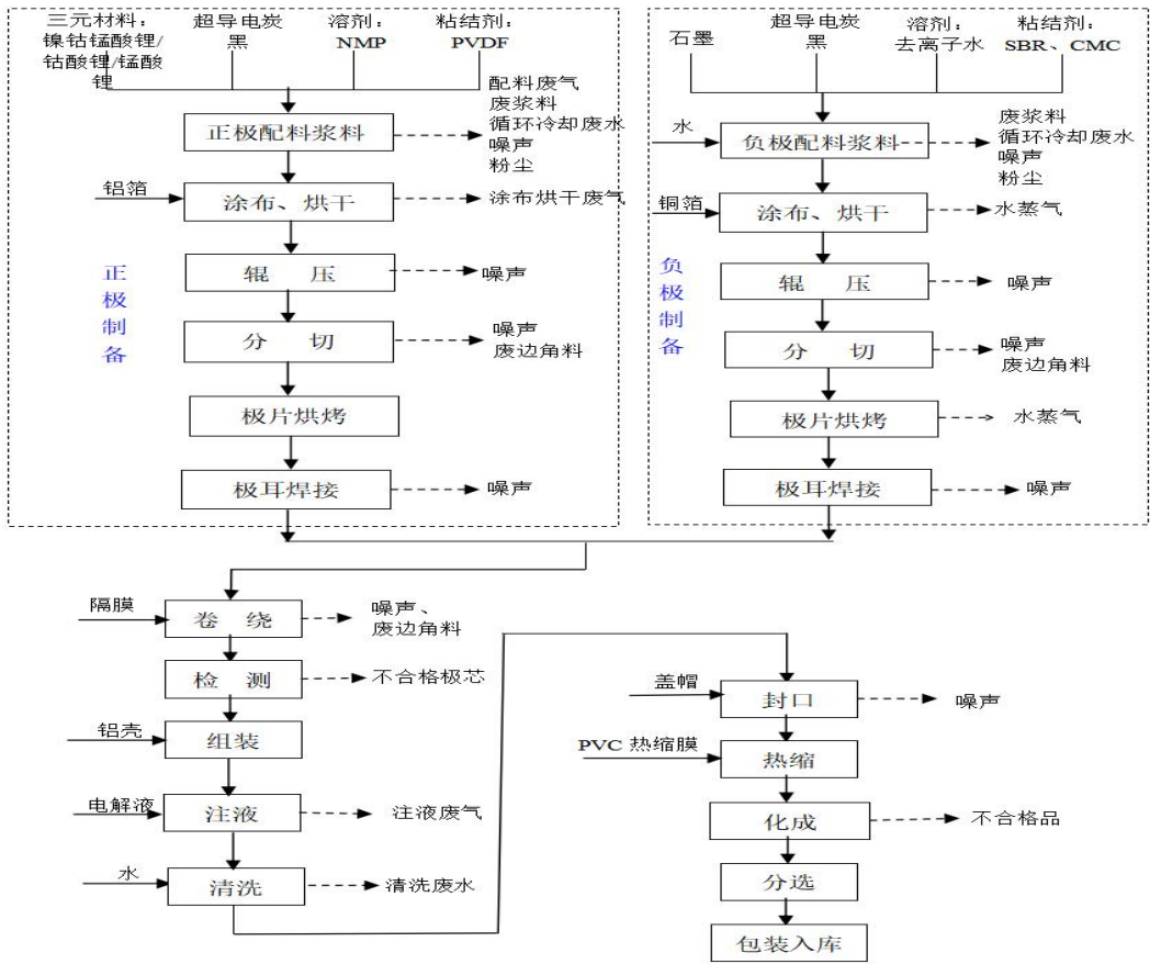
图 2-3 锂电池生产工艺
